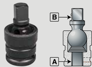
Giunto universale
