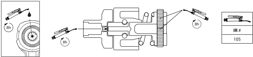
(Desenho TL-W7153-PIM-2)
